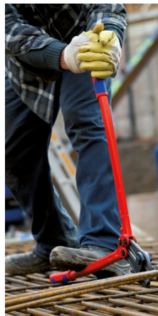
Gesmede aanslag met dempingsinzetstuk: dempt de snijslag comfortabel
